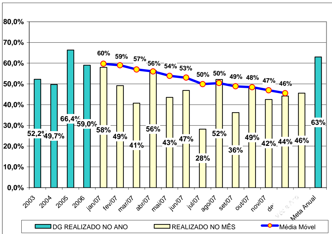
Gráfico 3 – Disponibilidade Geral da CGTEE – Período 2003 a 2007
