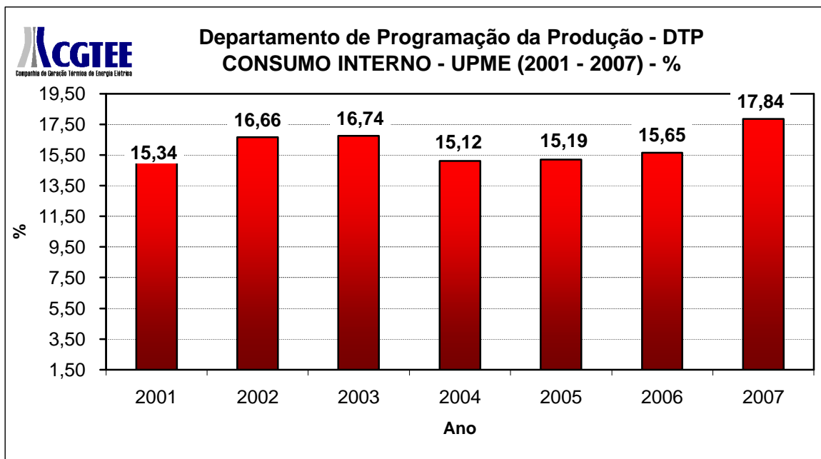
Gráfico 13 - Consumo Interno da UPME.
