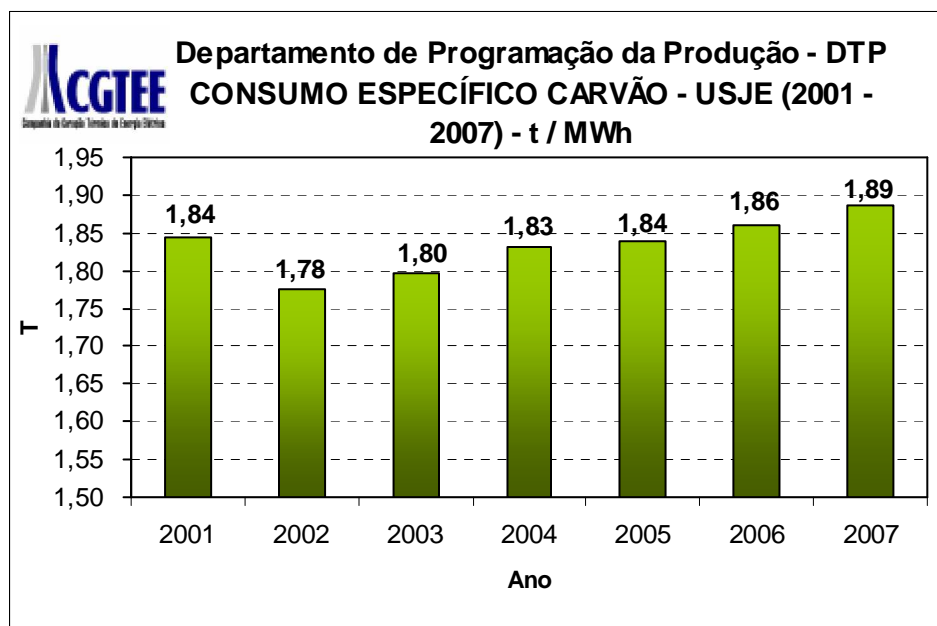
Gráfico 6 – Consumo específico de carvão na USJE.
