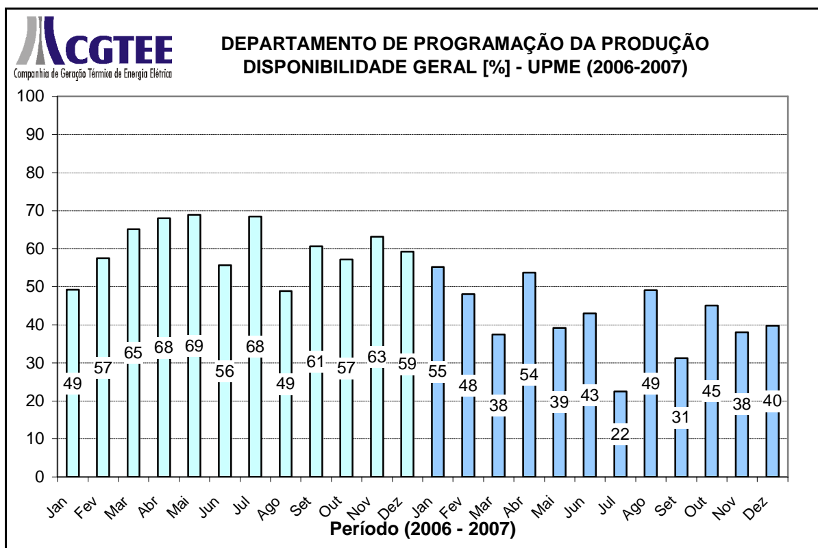
Gráfico 14 – Disponibilidade mensal do biênio 2006-2007.
