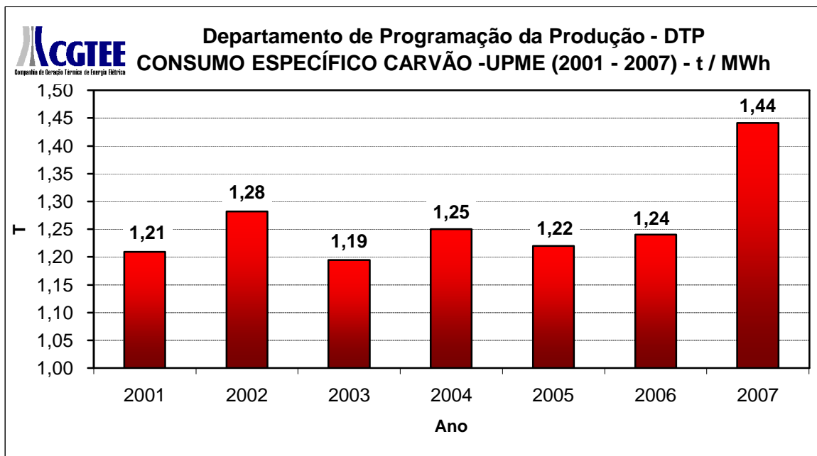
Gráfico 12: Consumo específico de Carvão 2001-2007 na UPME.
