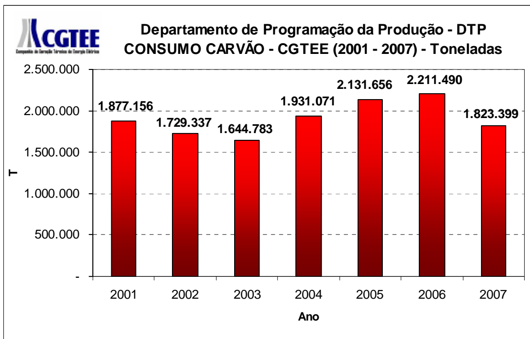
Gráfico 4 – Consumo de carvão na CGTEE no período de 2001 a 2007.
