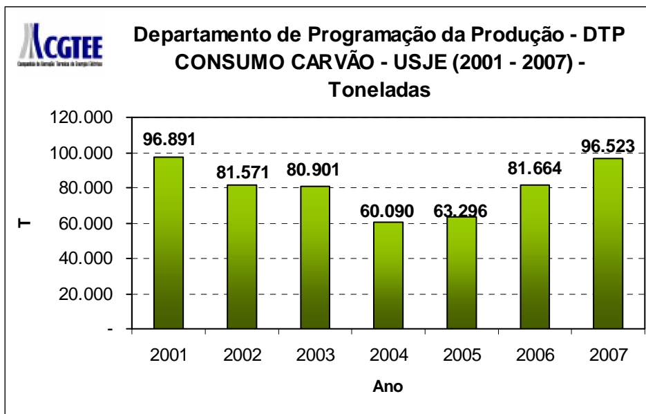
Gráfico 5 – Consumo de carvão na USJE
